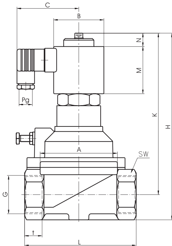
Maßzeichnung Standardausführung Dimensional drawing of standard type
